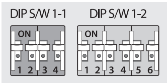
Main PCB Dip 스위치
